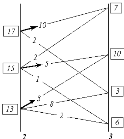
OBĽ. 9. K PODSTATE MDP. ANALÝZA PRECHODOV.
