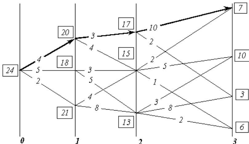
OBRAZ 10. K PODSTATE MDP. — OPTIMÁLNA TRAJEKTÓRIA.
