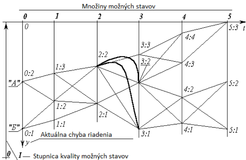
OBR. 11. DYNAMICKÉ PROGRAMOVANIE, ROZLIŠENIE A DVTR
