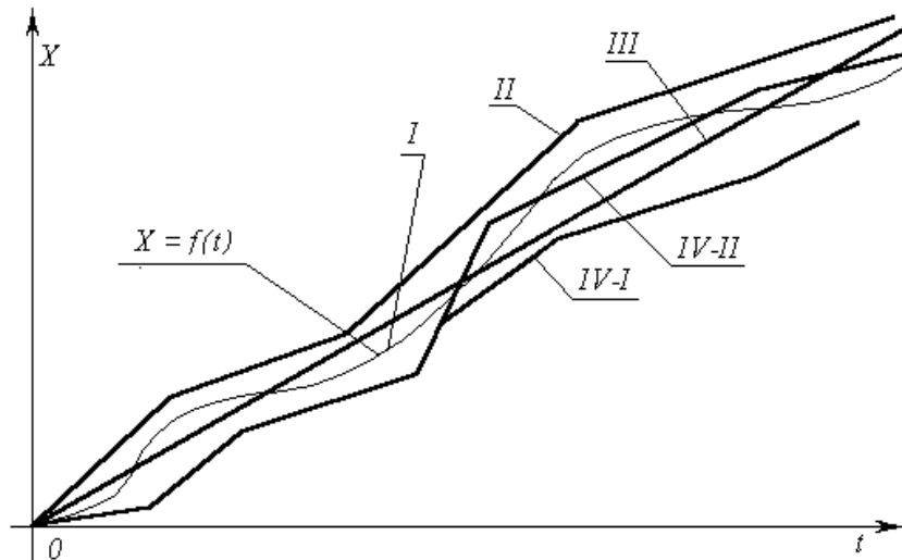
OBR. 4. NELINEÁRNY PROCES A JEHO LINEÁRNE OPISY.
