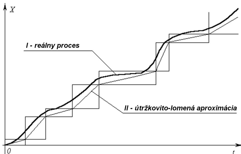
OBR. 5. LINEÁRNE APROXIMÁCIE A DISKRÉTNY CHARAKTER VÝPOČTU A KONTROLY PARAMETROV RIADENÉHO OBJEKTU.
