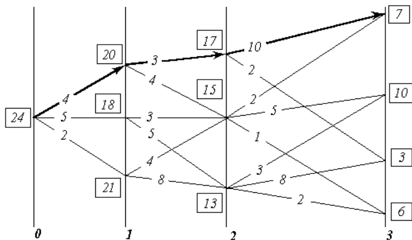
OBR. 8. K PODSTATE METÓDY DYNAMICKÉHO PROGRAMOVANIA.
