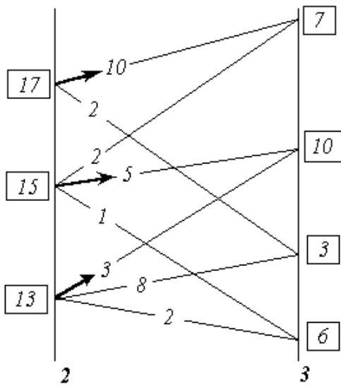
OBR. 7. K PODSTATE METÓDY DYNAMICKÉHO PROGRAMOVANIA
