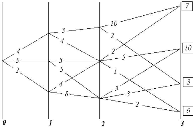
OBR. 6. K PODSTATE METÓDY DYNAMICKÉHO PROGRAMOVANIA
